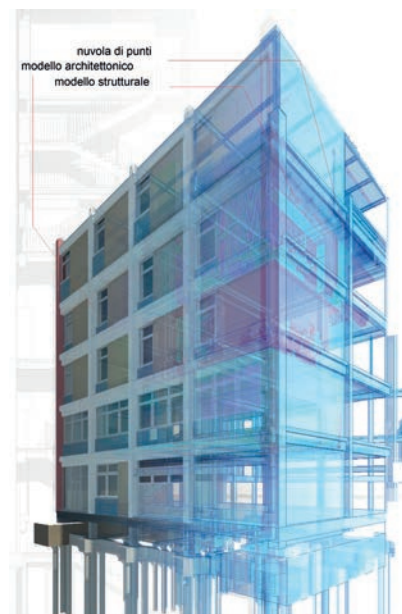
Procedura Scan to Bim: dal rilievo 3D alla modellazione informatizzata per la progettazione degli interventi di riqualificazione energetica e funzionale del complesso edilizio dell'Università degli Studi di Napoli Federico II
